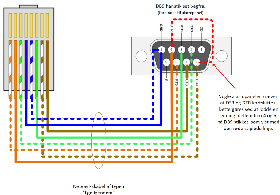
Serielt kabel - RJ45 - DB9 han
