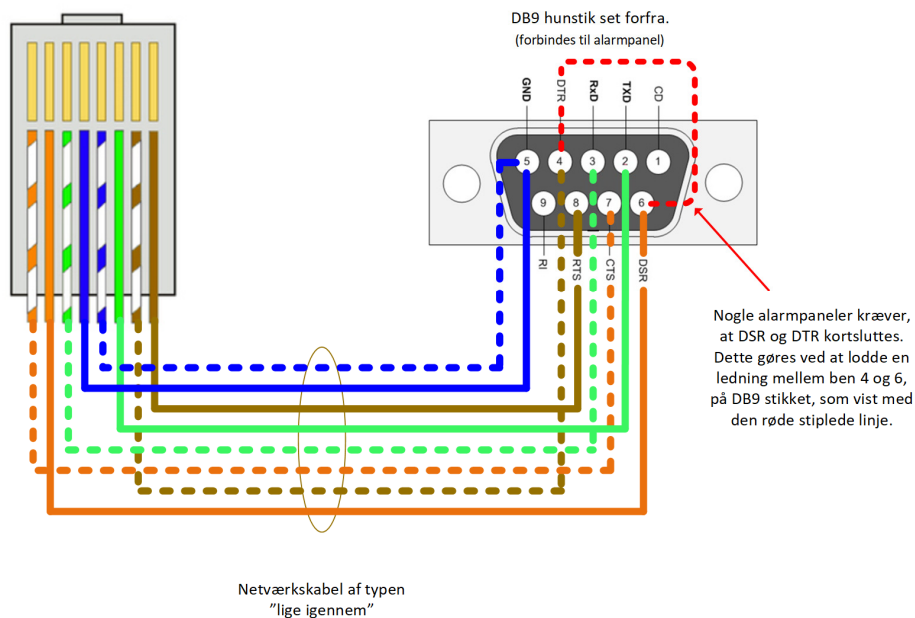
Serielt kabel - RJ45 - DB9 hun
